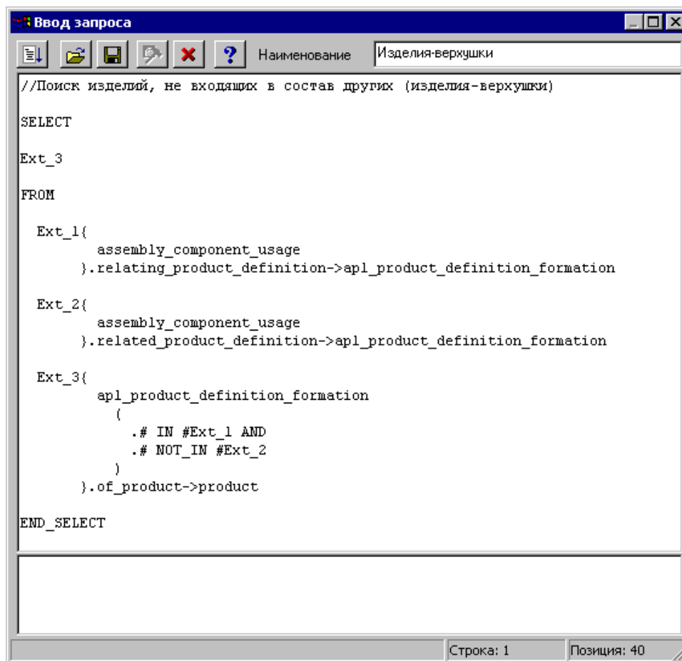
Рисунок 2.21. Окно редактора запросов на языке STEPQL
