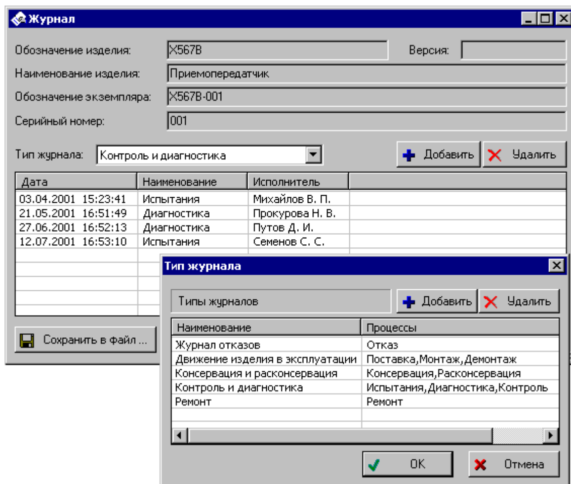
Рисунок 2.19. Диалоговое окно модуля "Журнал экземпляра изделия"
