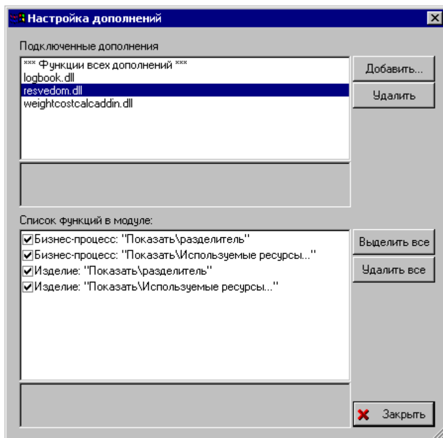
Рисунок 5.1. Окно подключению модулей дополнения
