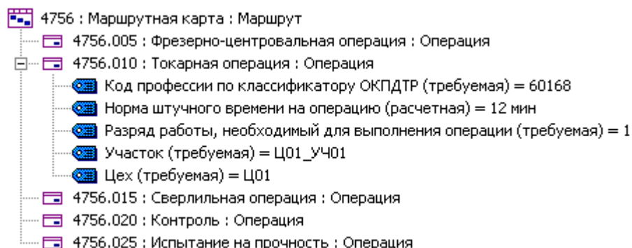
Рисунок 2.9. Пример характеристик БП-операции
