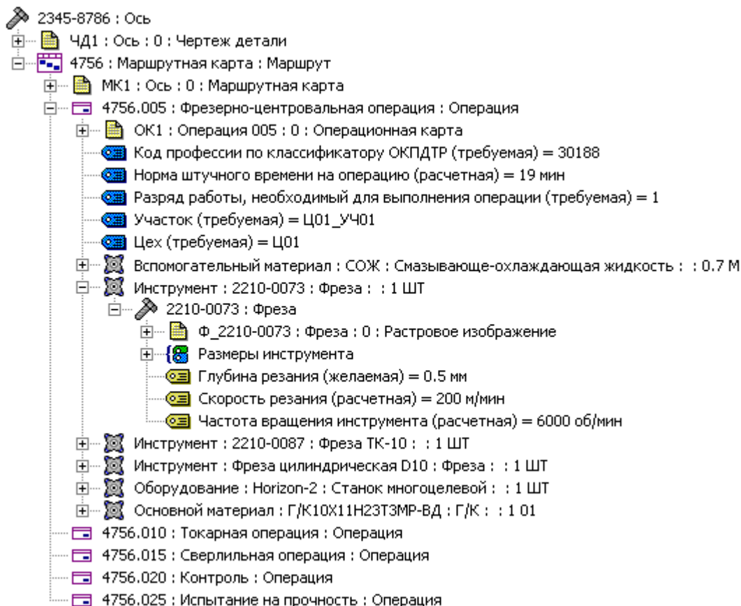
Рисунок 2.16. Пример технологической информации
