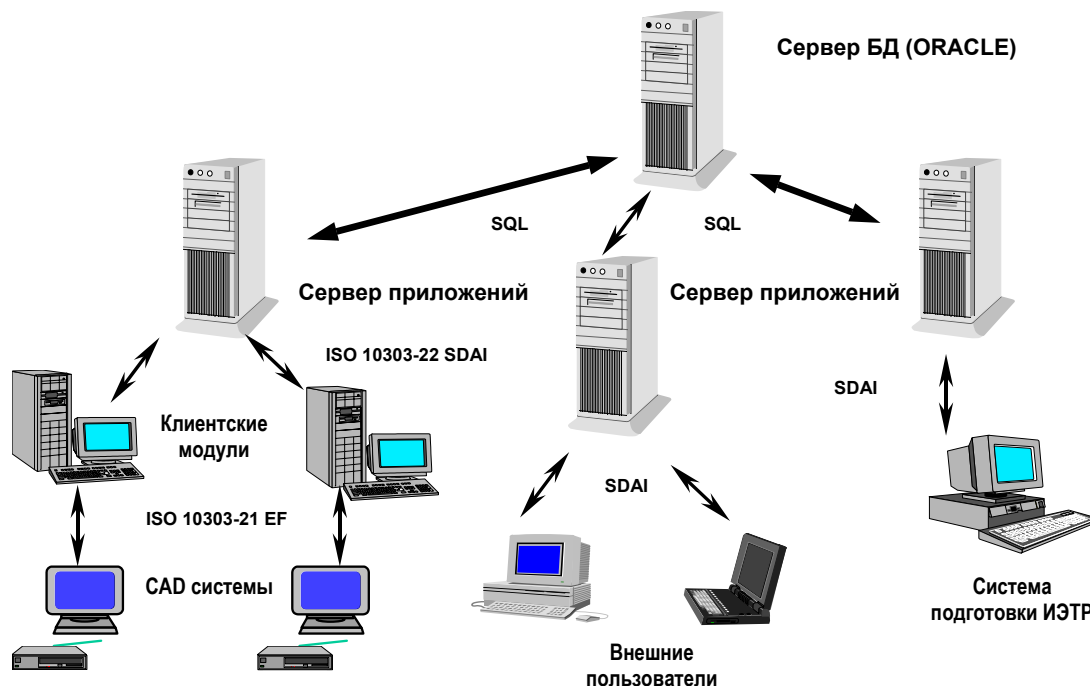
Рисунок 3.1. Трехуровневая архитектура "Клиент-Сервер"
