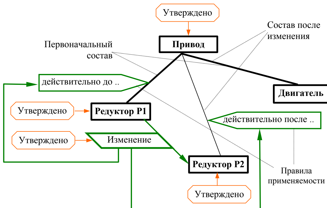
Рисунок 2.11. Описание изменения структуры изделия в PSS
