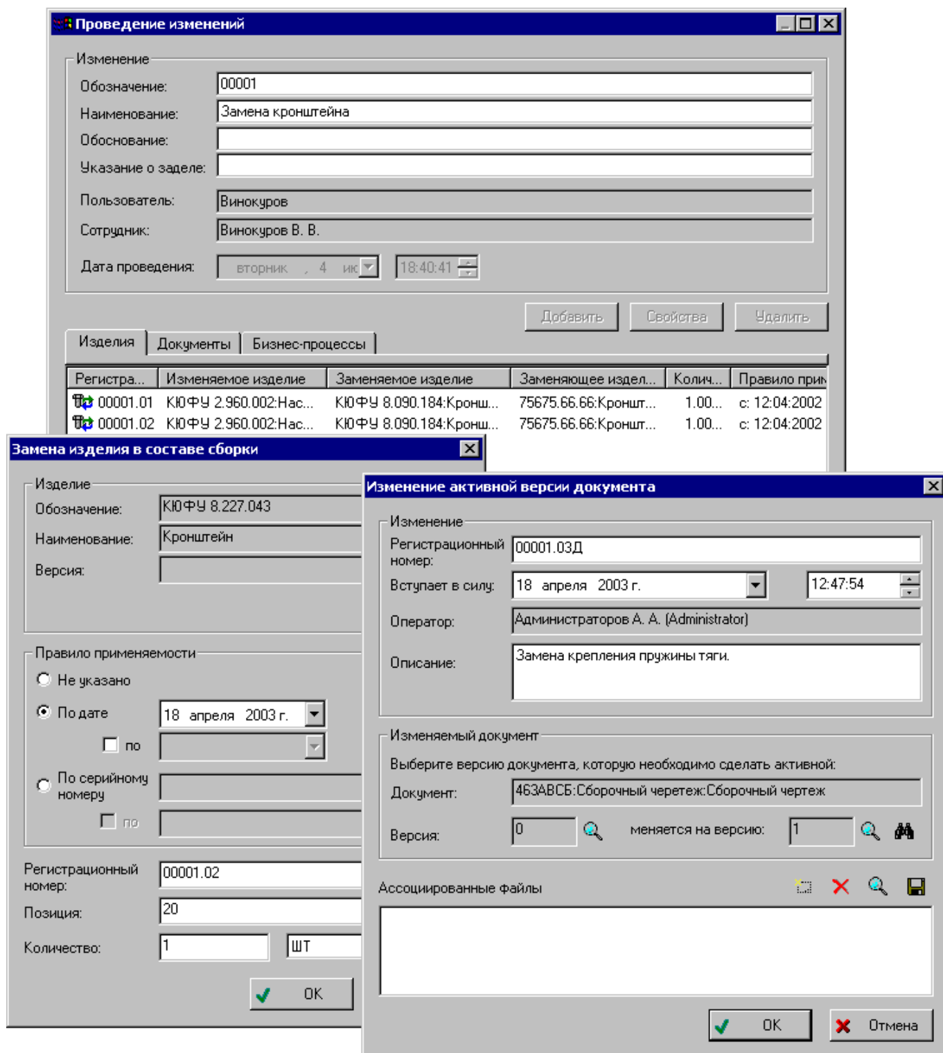
Рисунок 2.12. Основные диалоговые окна механизма изменения
