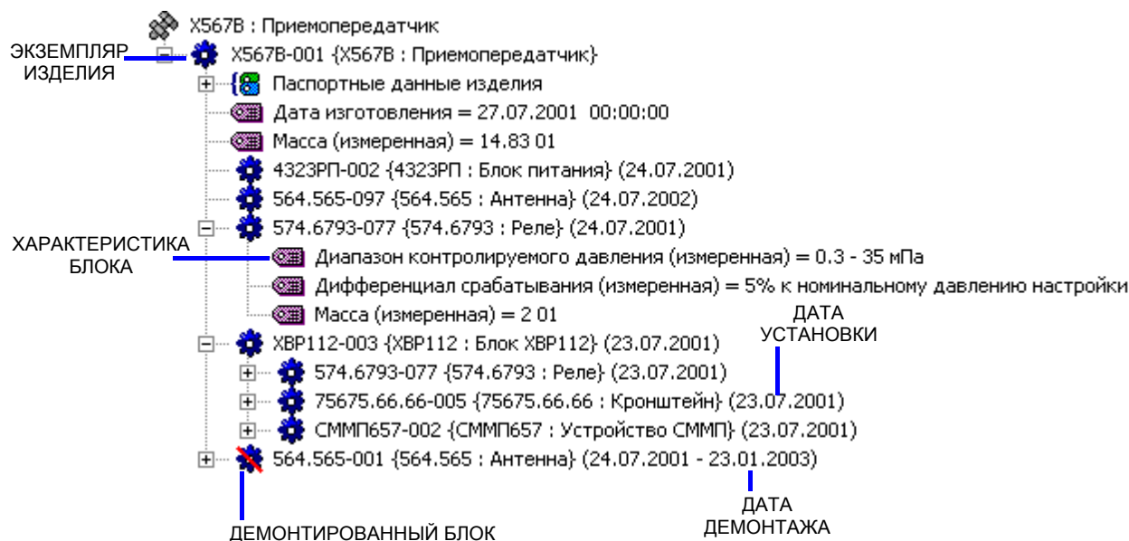
Рисунок 2.17. Пример экземпляра изделия
