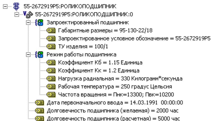
Рисунок 2.8. Пример характеристик версии изделия
